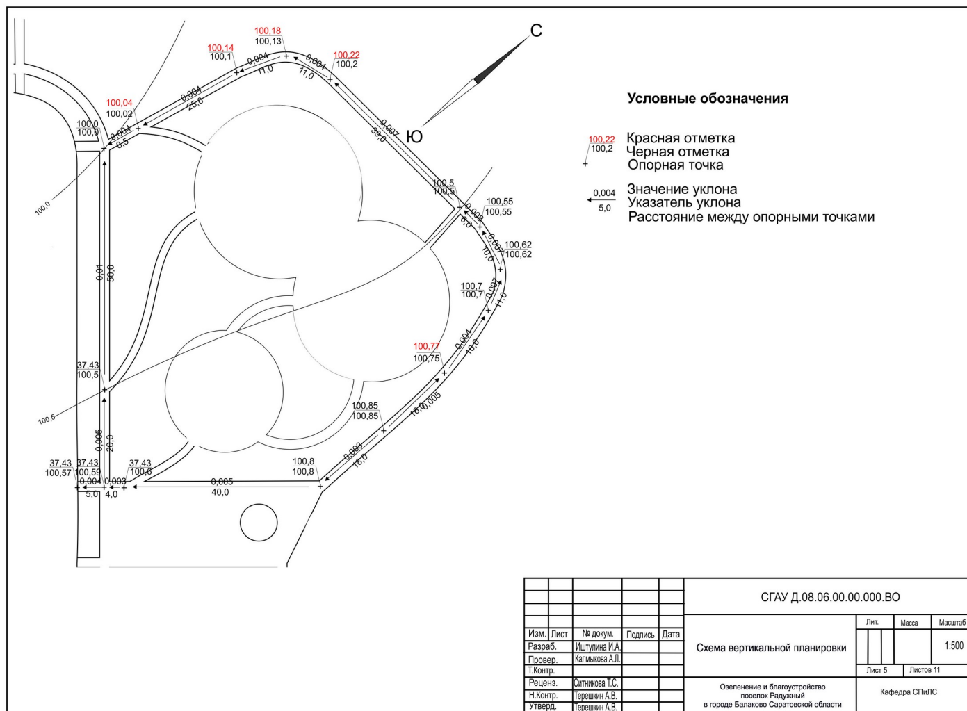
Схема вертикальной планировки в проектных отметках.
