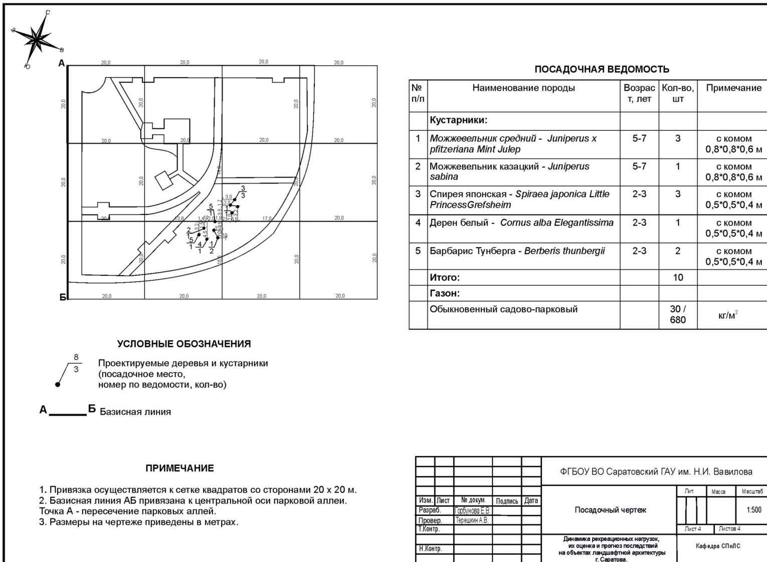
Посадочный чертёж
